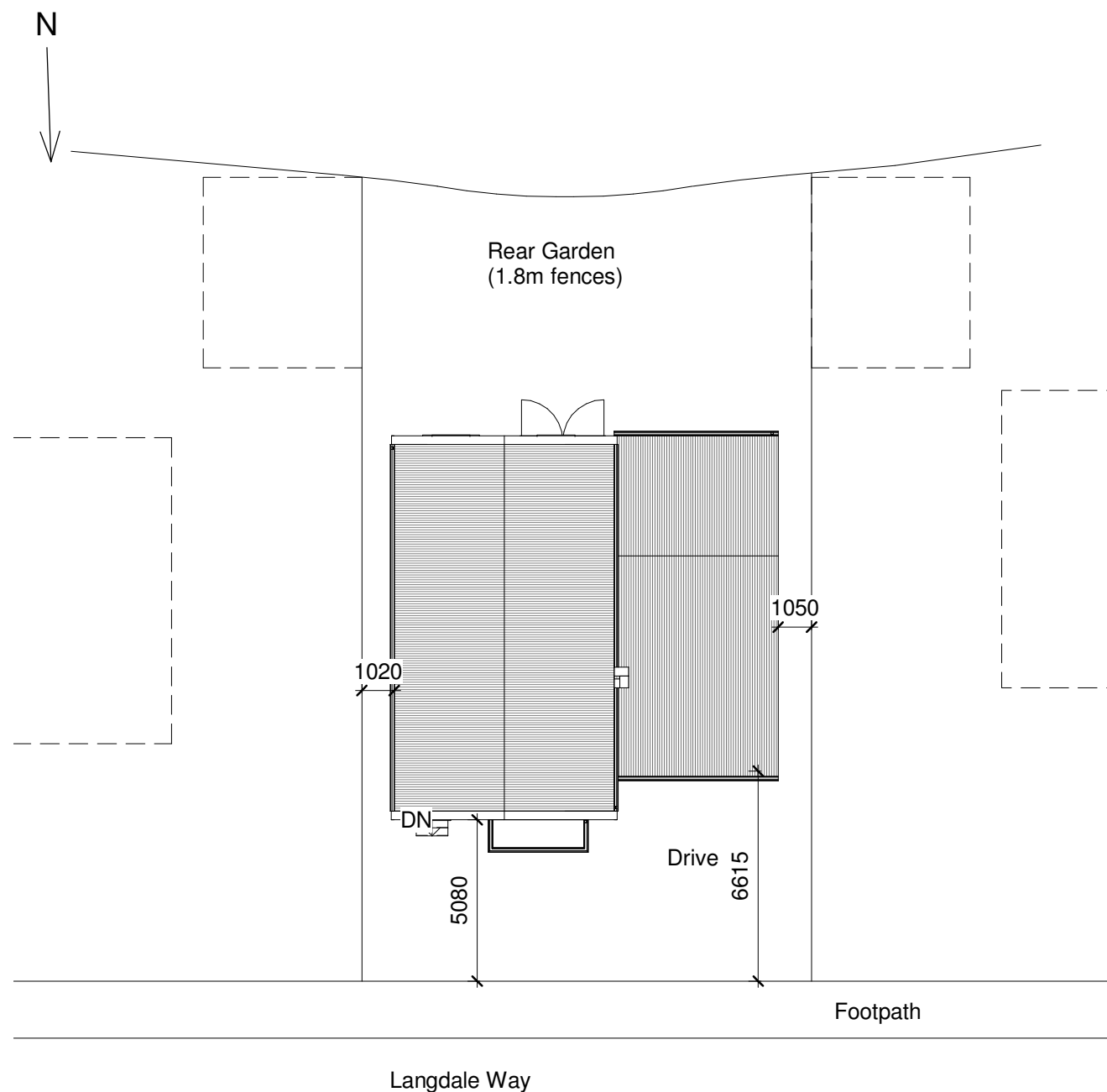
1 Site 1 : 200
